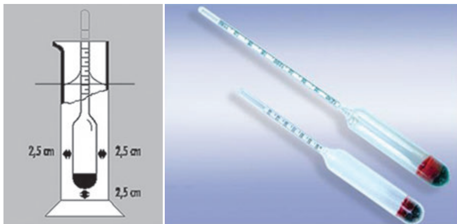
Рисунок 1. Прибор для измерения плотности приготовленных растворов солей.
