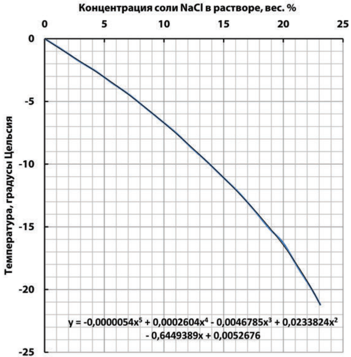
Рисунок 4. Кривая замерзания водных растворов хлорида натрия (NaCl), построенная по данным, приведенным в кратком справочнике химика, издательство «Химия», М-Л, 1964 г.
