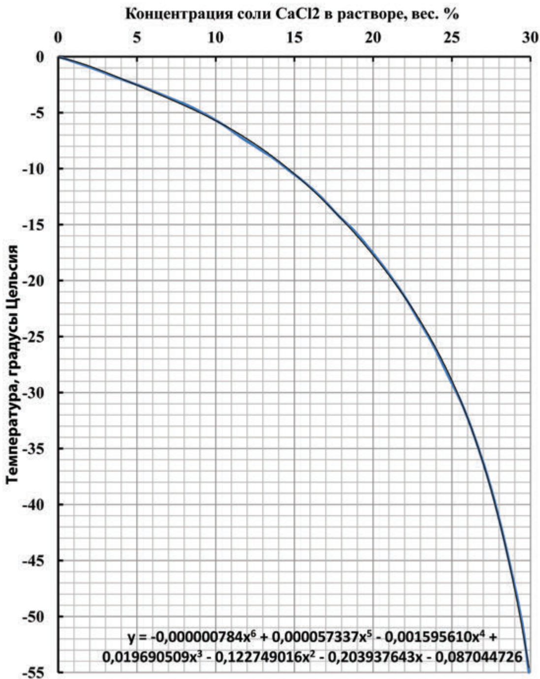
Рисунок 5. Кривая замерзания водных растворов хлорида кальция (CaCl 2 ), построенная по данным, приведенным в кратком справочнике химика, издательство «Химия», М-Л, 1964 г.
