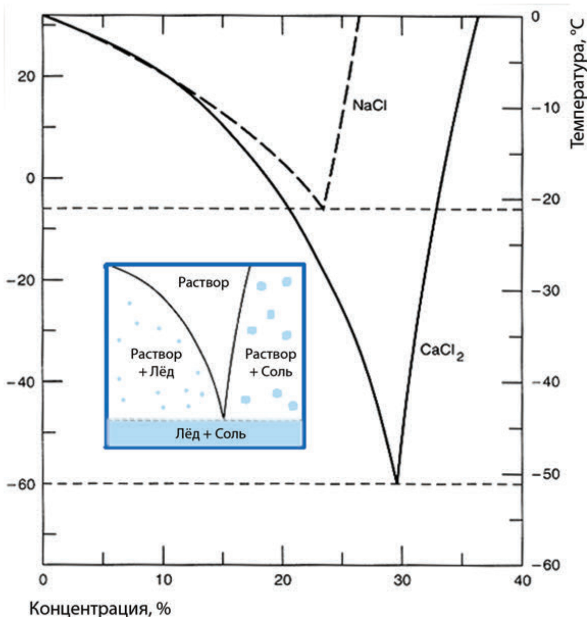
Рисунок 3. Кривые замерзания (фазовые диаграммы) растворов хлористого натрия и хлористого кальция.
